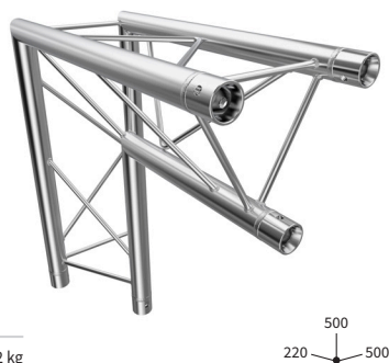
90° ECKE | CORNER C25 CODE F23C25
