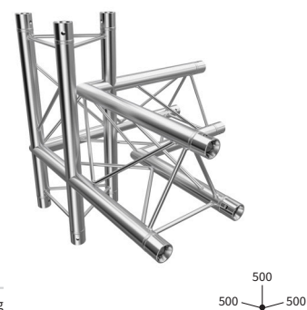
4-WEG ECKE | 4-WAY CORNER C45 CODE F23C45
