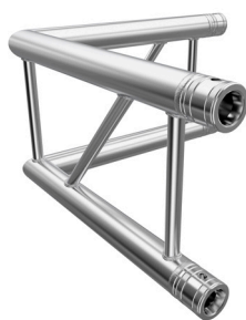
90° ECKE | CORNER C21V CODE F32C21V
