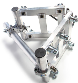
VARIABLE ECKE | CORNER 0-180° Der Winkel ist nur von ca. 20° bis 75° mit der mitgelieferten Stange arretierbar. CODE F34VC0-180
