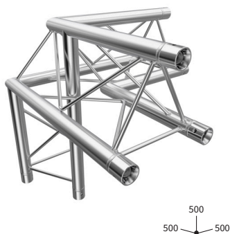
3-WEG ECKE | 3-WAY CORNER C32 CODE F23C32
