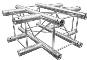
4-WEG ECKE | 4-WAY CORNER C41 CODE F24C41
